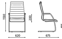
LYNX LB CFP-CR Gewicht: 16,6 kg
